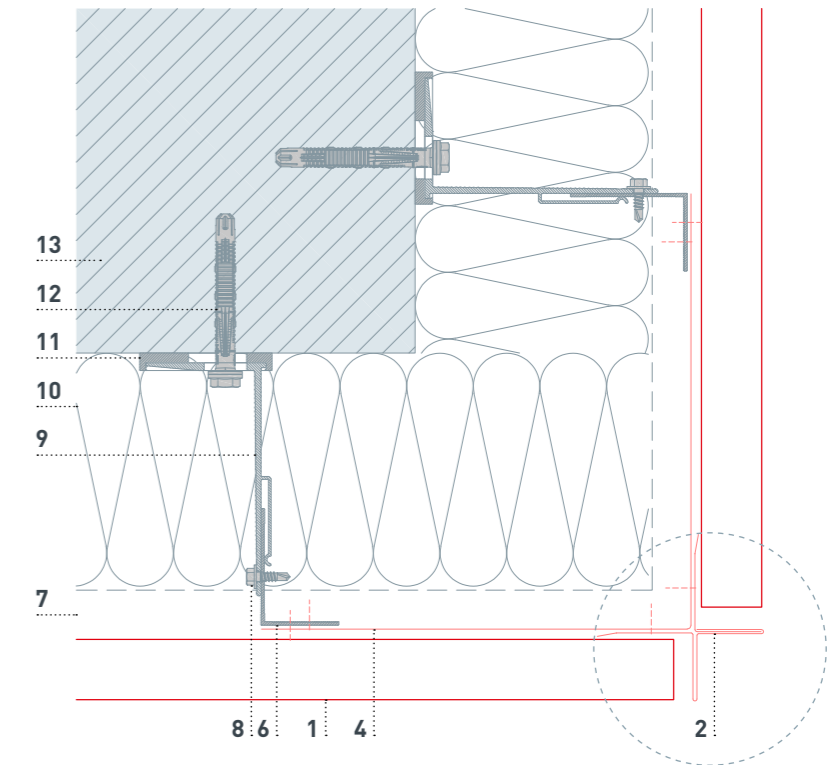
variante de raccordement
