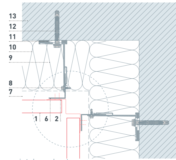
variante de raccordement
