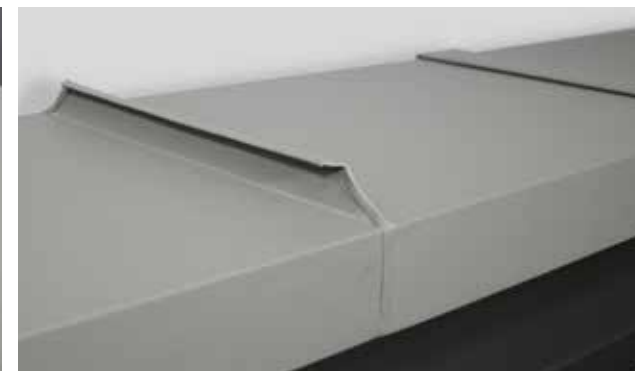
staande naad
