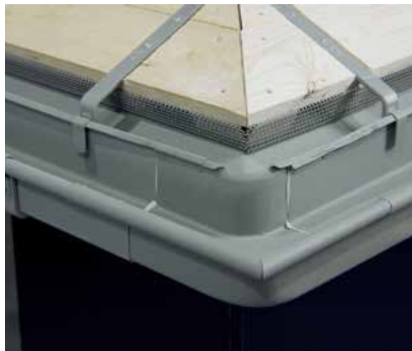
buitenhoek goot
