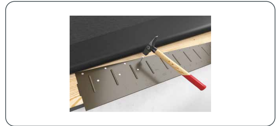
Abbildung 54 • Saumstreifen
