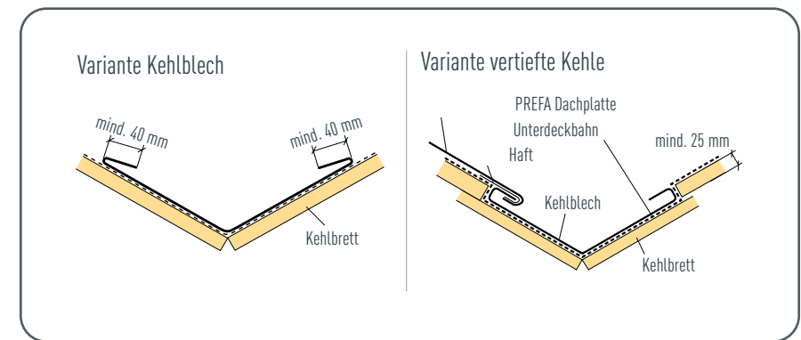
Abbildung 59 · Varianten Kehlblech und vertiefte Kehle
