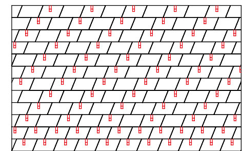
VERLEGESCHEMA DS2
