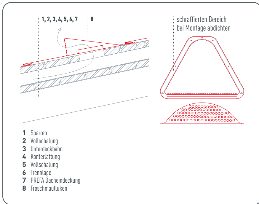
Abbildung 119 · Froschmaulluke
