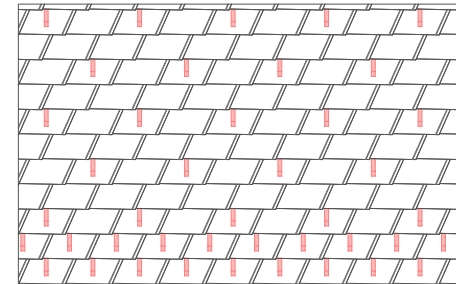
VERLEGESCHEMA DS.19 1
