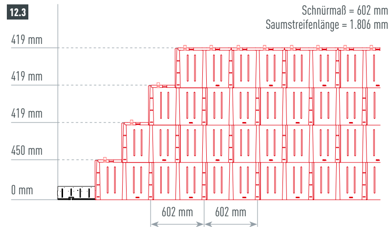
Abbildung 12 • Dachplatte – Schnürmaß
