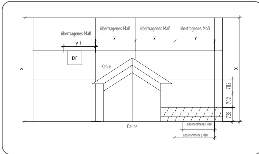
Abbildung 23 • Dachschindel – Schnürung
