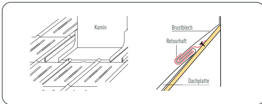
Abbildung 104 • Kamineinfassung – Dachplatte
