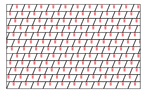
Abbildung 77 • Verlegeschemen mit dem Schneestopper für die Dachschindel
