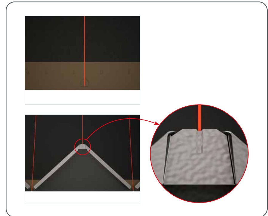
Abbildung 35 · Dachraute 29×29 – Schnürmaß
