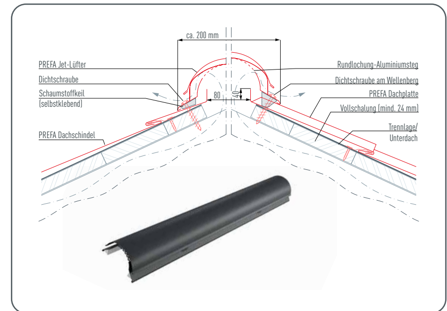
Abbildung 62 · Jet-Lüfter
