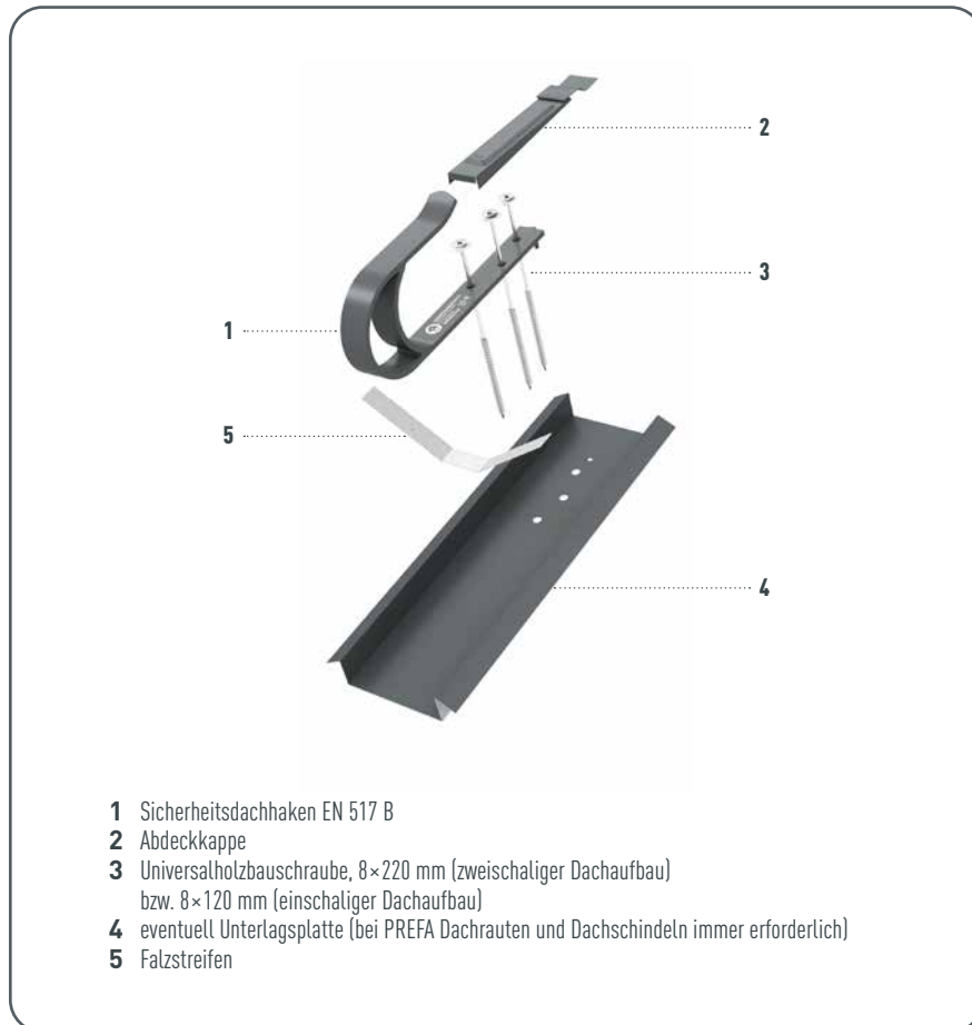
Abbildung 102 · Sicherheitsdachhaken – Benötigtes Material
